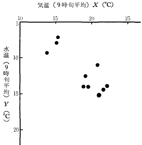
図 16 気温 (9時旬平均) と水温 (9時旬平均) との相関図 (33年度 溢水終点)
