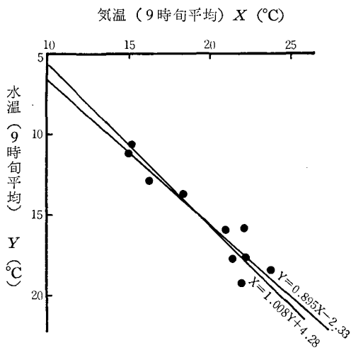
図 24 気温（9 時旬平均）と水温（9 時旬平均）との相関図 （34 年度 池壳取水口）
