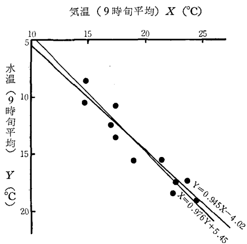
図 23 気温（9 時旬平均）と水温（9 時旬平均）との相関図 （34 年度 発電所放水口）
