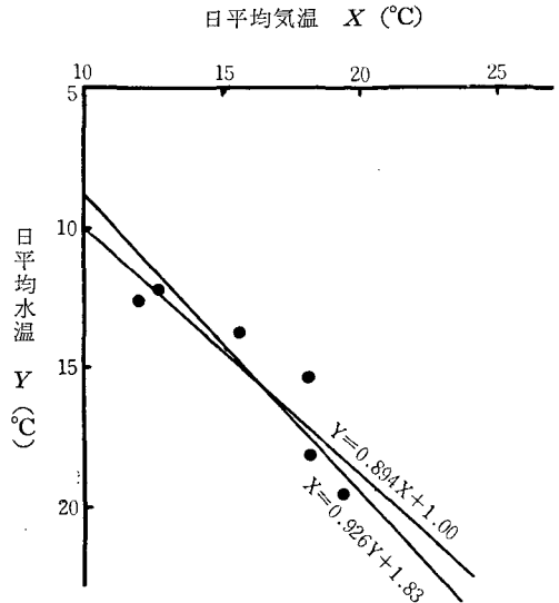
図 15 日平均気温と日平均水温との相関図 (34年度 長知内取水口)
