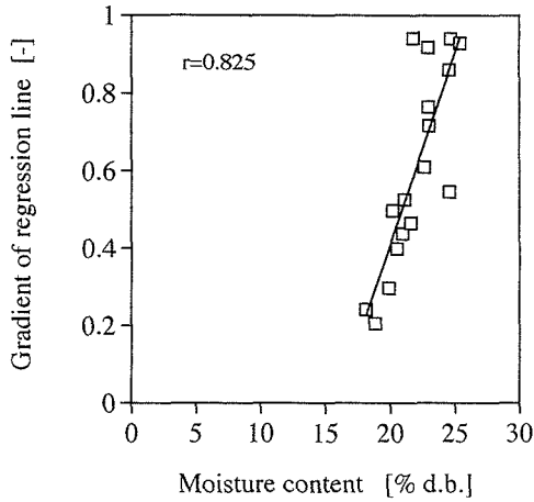
図 4.8 土壤含水比と土塊亀裂の大きさの回帰直線の傾き
