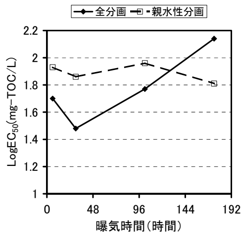
図-1 長時間曝気活性汚泥試料の LogEC 50 値の経時変化
