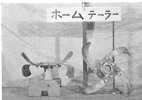
Fig. 4. Knife Rotor.
