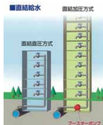
図2 直結給水方式
