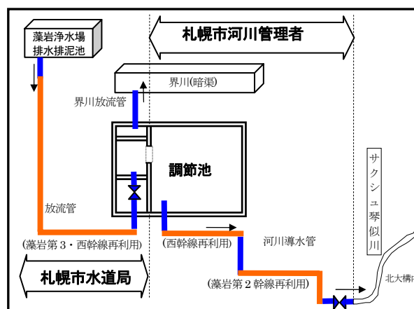
図3 サクシュ琴似川導水施設
