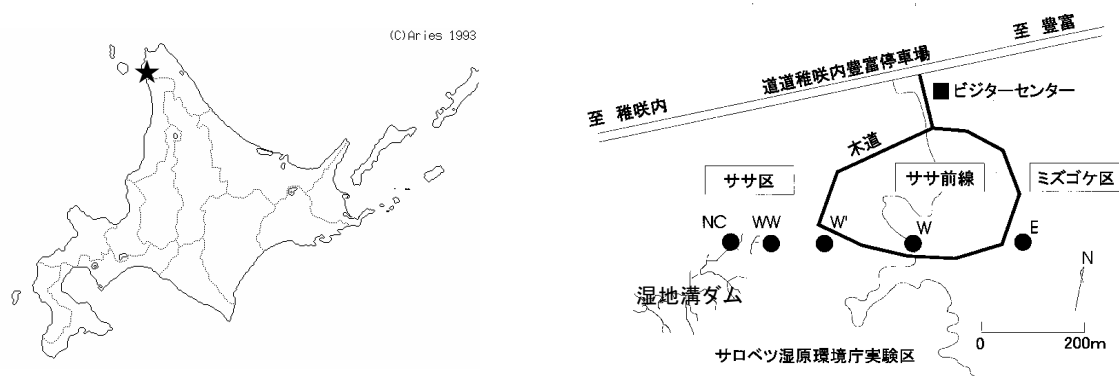
図1 サロベツ湿原の位置と調査地点の概況
