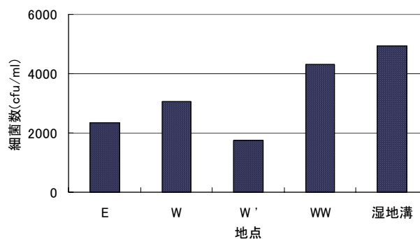
図2 好気性細菌数(03年10月)
