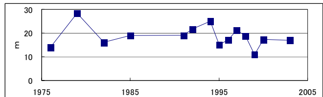
図 5.COD の経年変化
