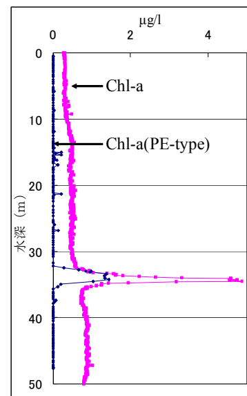
図 7.Chl-a と Chl-a (PE-type) の鉛直分布
