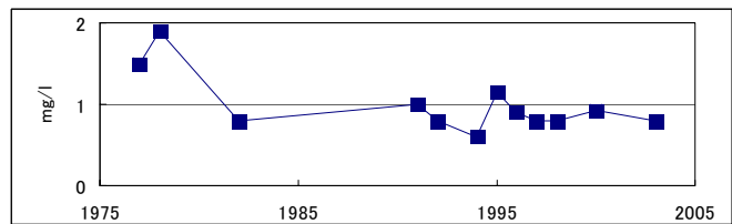
図 4.透明度の経年変化
