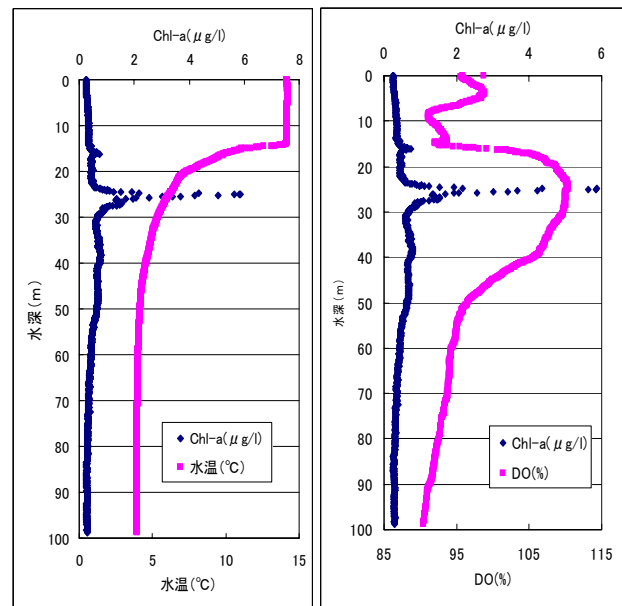
図3 クロロテックと水温（左）、DO（右）の関係（2003年7月23日）
