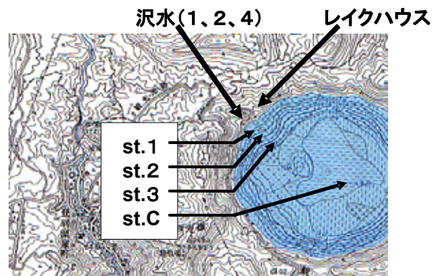
図2. 採水地点
