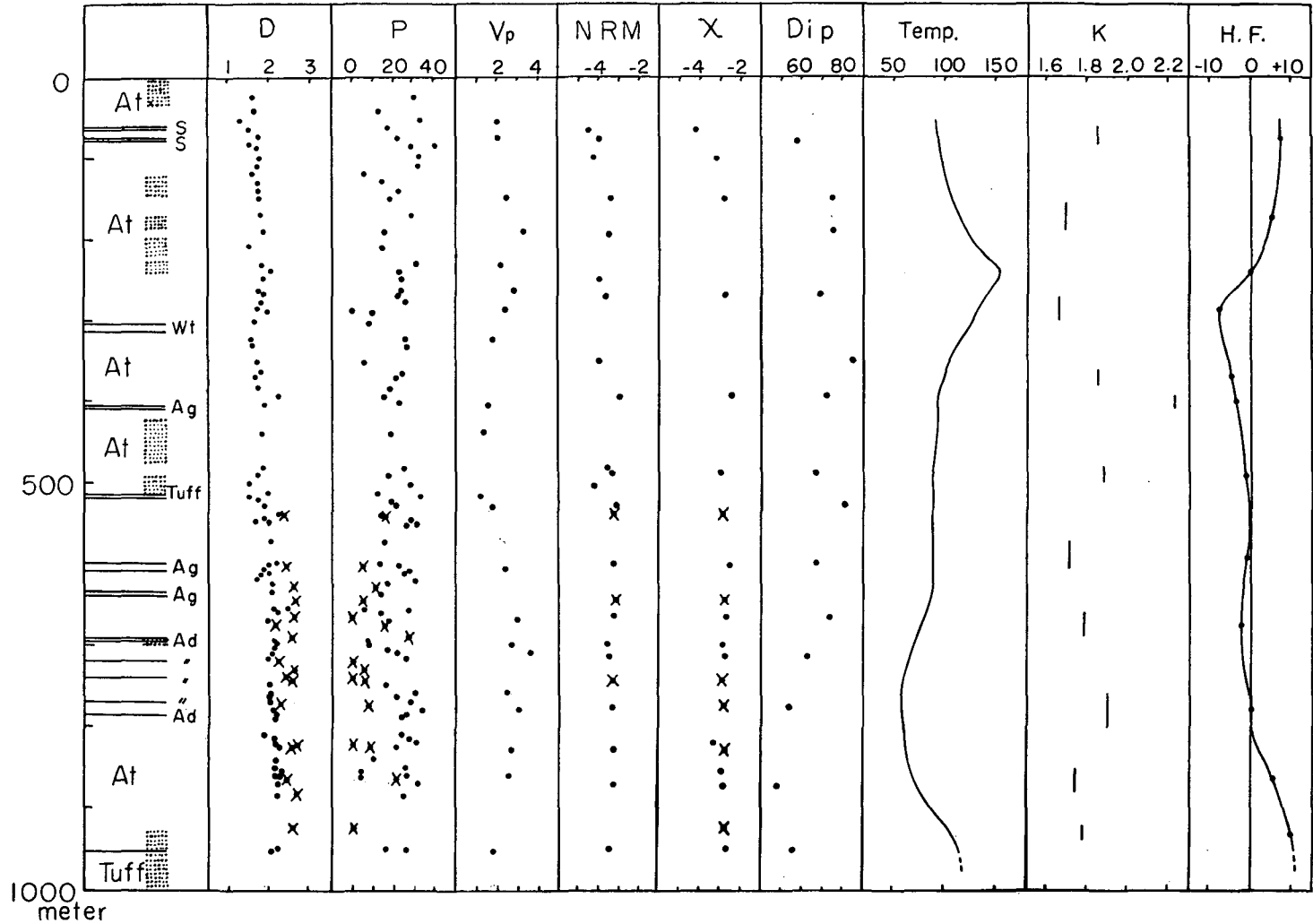
第2図 測定結果
