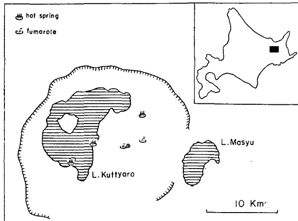
第1図 屈斜路カルデラ (◎印はボーリング位置)
