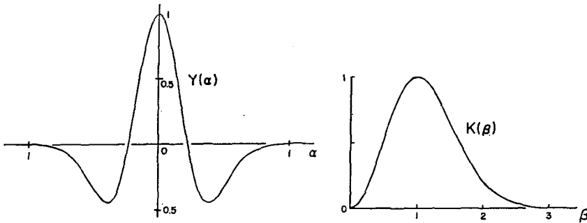
第2図 RICKER の wavelet とその FOURIER 変換 Fig. 2. RICKER's wavelet and its FOURIER transform.
