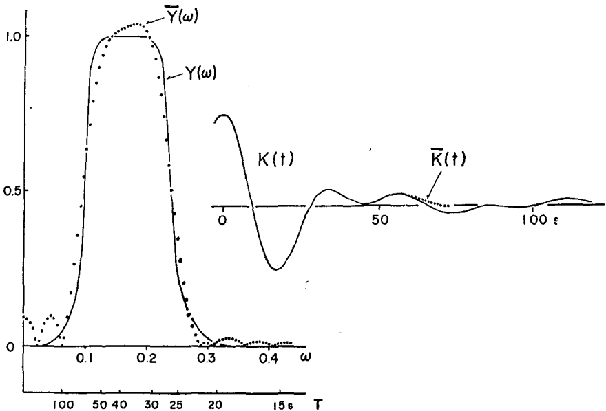
第1図 計画された特性と実際の特性, およびそれらの衝撃応答
