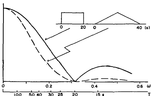
第3図 移動平均および二重の移動平均の特性
