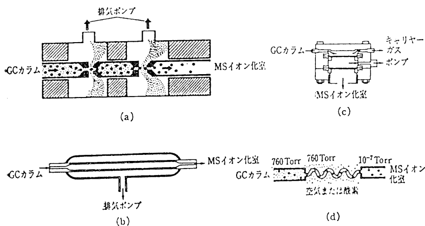
図 7-4 代表的なセパレーター
