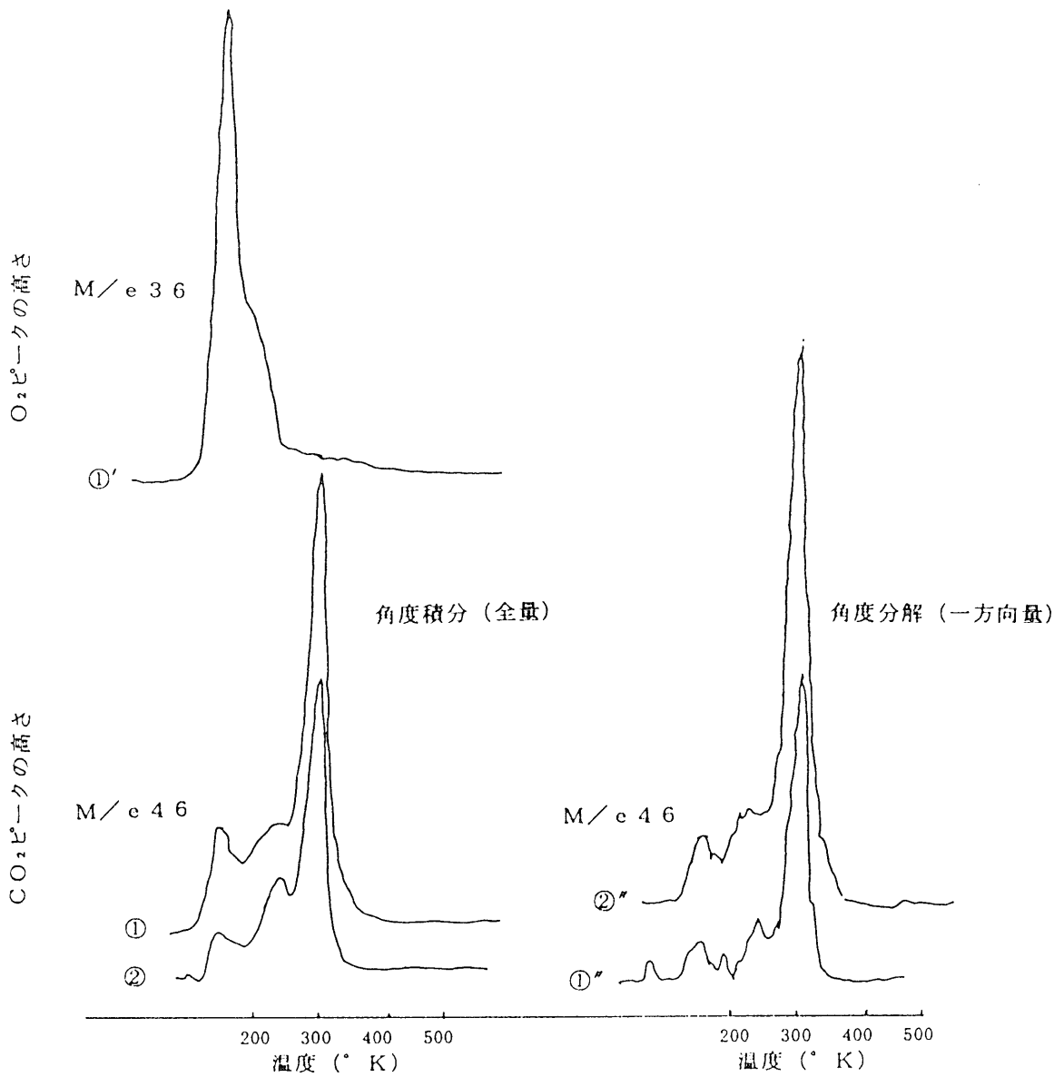
図11 MSによるCO 2 脱離ピークの変化
