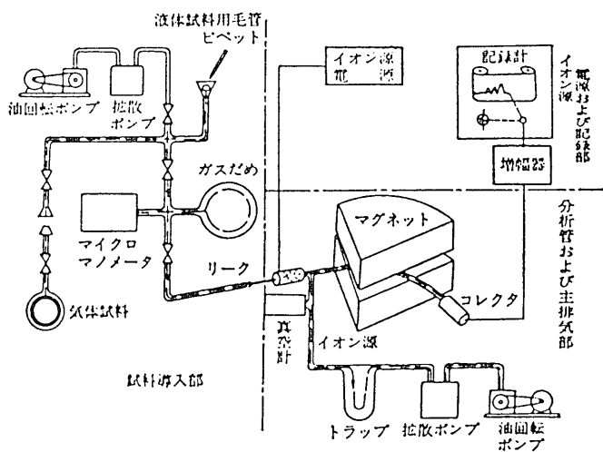
図2 質量分析計の配置図
