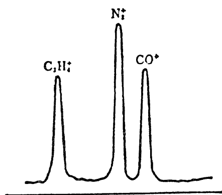
CO, N 2 , C 2 H 4 の分離
