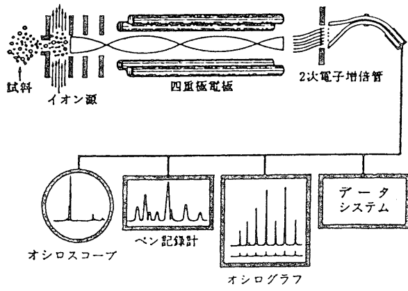
図9 4重極質量分析計概略図
