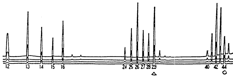
図3 エタノールとアセトアルデヒドのMSスペクトル
