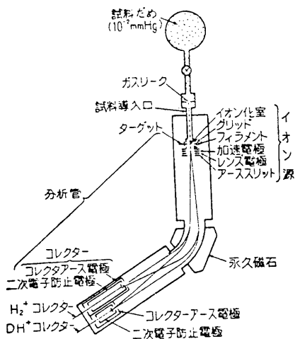
日立 RDM-3 型重水素用質量分析計原理図
