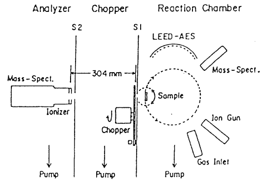
図10 表面分子ダイナミクス部門での 超高真空装置の概略図
