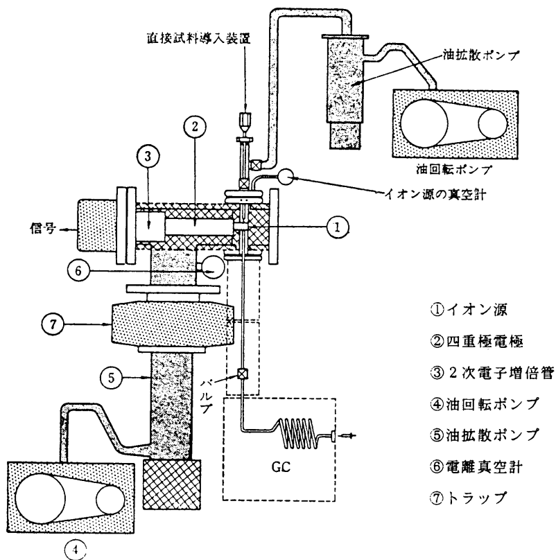
図8 4重極質量分析計の基本構成と配置
