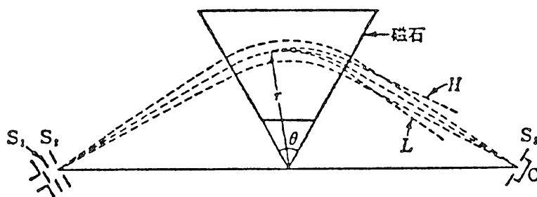
図1 単収束磁場偏向型質量分析計原理図
