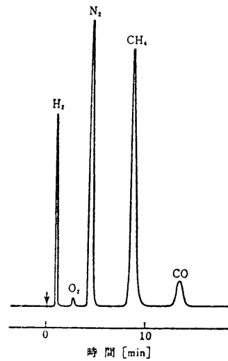
図7 GCのクロマトグラム
