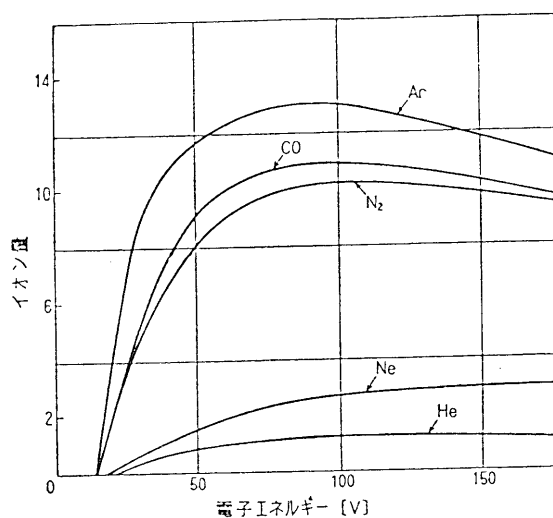
図5 イオン化効率曲線
