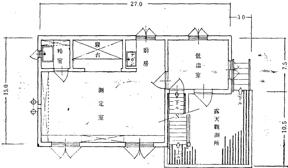
—— 主階平面 ——
