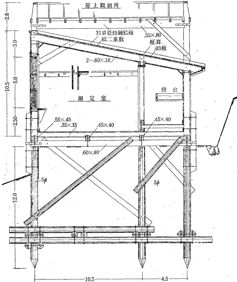
第 4 圖 家の構造断面圖
