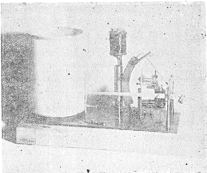
(寫眞2) 自記霧水量計第2號
