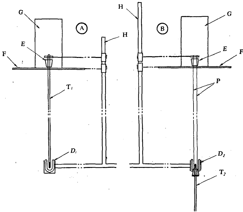
第 2 圖 装置 A 及び B の略圖
