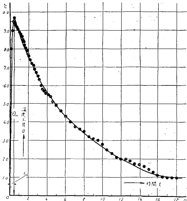
第4圖 小 Dewar's vessel についての水、硫酸混合後の溫度上昇と時間經過との關係 (黒丸は實測の1例)
