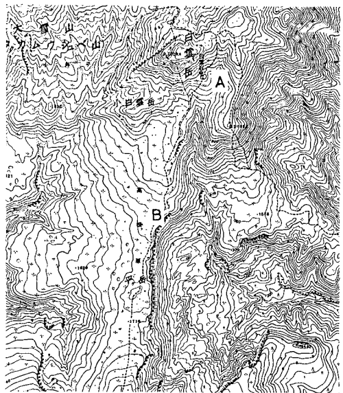
第4図 大雪山系白雲岳周辺図 Aはポリゴン観測点, Bは高根ヶ原気象観測地点
