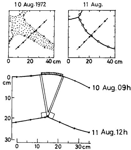
第17図 ゴミの移動の観測例 (X=16, Y=10の地点) 上2図は平面図、下は平面図中1点鎖線部分の垂直断面図
