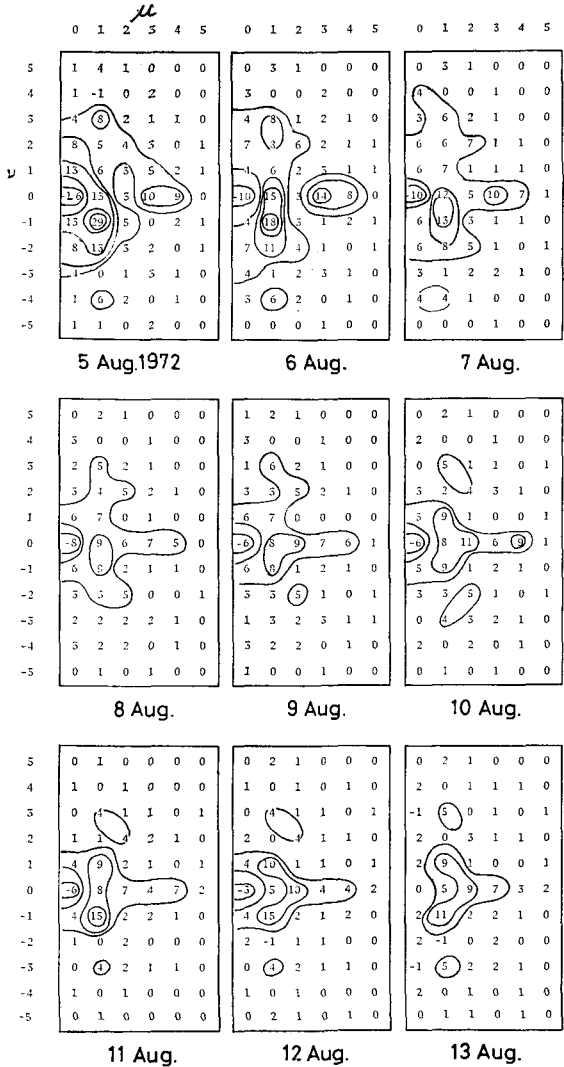
第10図 ポリゴンのパワー・スペクトルの変化
