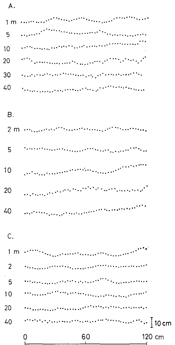
第18図 雪渓 No. 1 の雪面の凹凸状況 A, B, C は第2図の A, B, C に対応、左の数字は雪渓の端からの距離を示す
