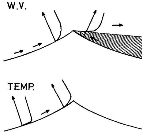
第 22 図 ポリゴンの上の風速・温度の垂直分布の考察
