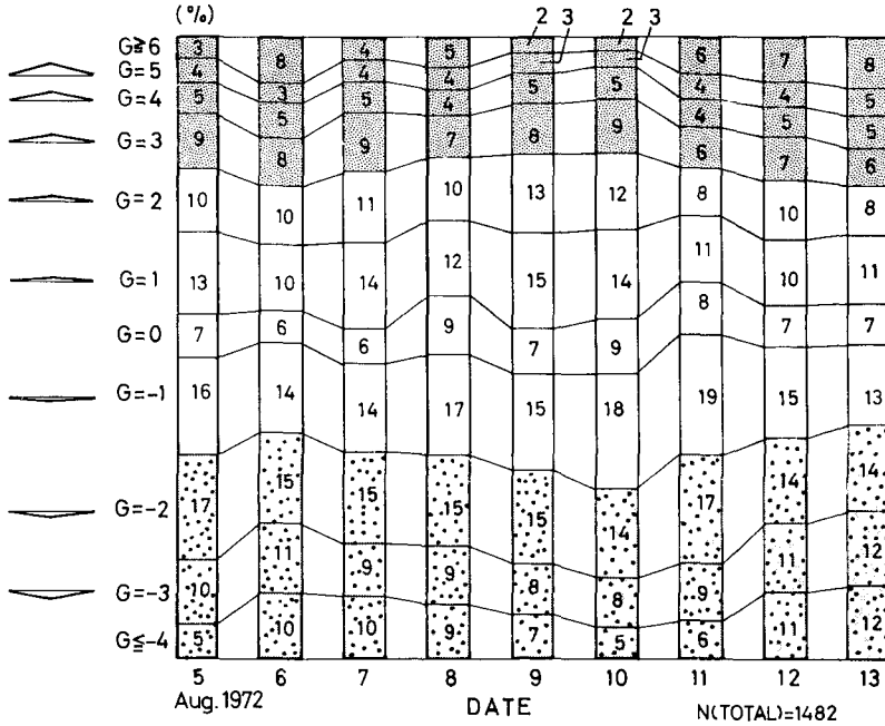
第7図 ポリゴンの尖度の度数分布の変化
