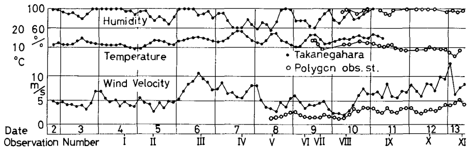
第5図 ポリゴン観測期間中の気象条件。●印は高根ヶ原、○印はポリゴン観測地点
