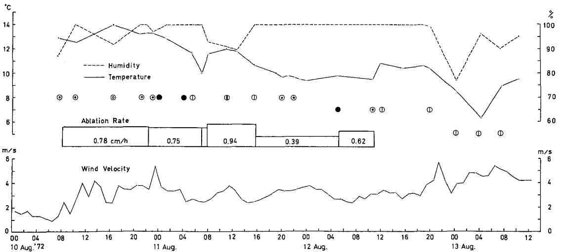
第13図 ポリゴン観測地点の気象条件および融雪速度
