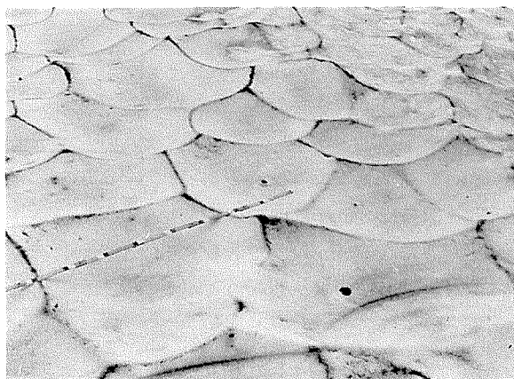
第1図 山岳地帯の雪渓上の亀甲模様 (ポリゴン) スケールの長さは1 m
