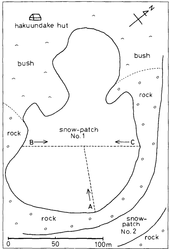
第2図 ポリゴンの観測地点 (大雪山系白雲岳東斜面の雪渓)
