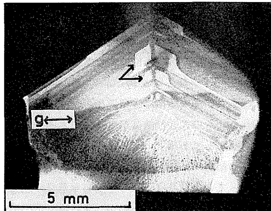
第1図 六角板結晶のX線トポグラフ走査面(0001)、反射面(10 \bar{1} 0)、試料とホルダーの接合部から転位が発生した
