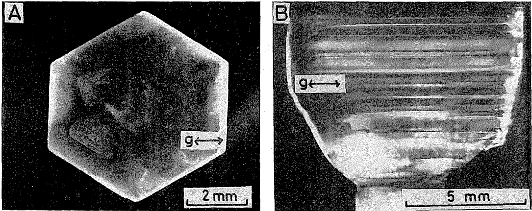
第3図 A: 六角板結晶。結晶の厚さは約0.7 mm, 中央左よりに層状の生長が見られる B: 四角形コップ型結晶の1片。反射面は(0002)面である
