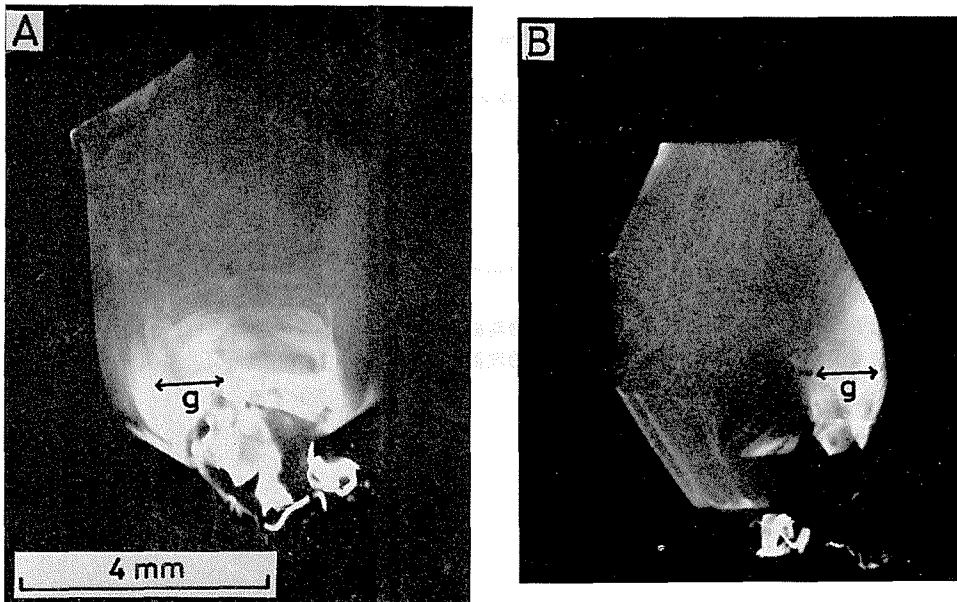
第4図 六角板結晶のX線トポグラフ。走査面はA, Bいずれも(0001)面, 反射面はAが (10\bar{1}0) , Bが (11\bar{2}0) である。Bの写真に転位が見られる
