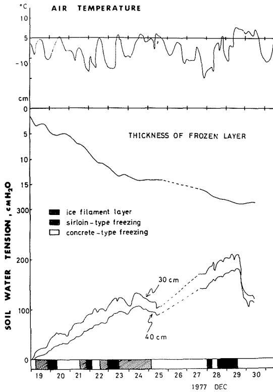
第2図 水分張力の変化と凍結型 (A プール)
