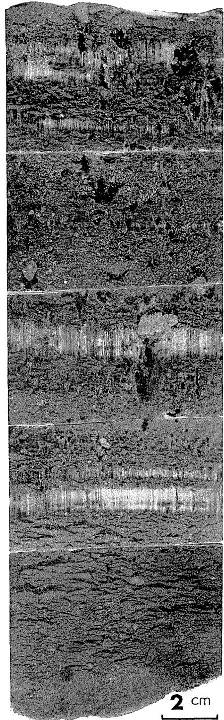
第3図 凍土の断面写真 (A プール) 写真の上面が地表面, 下面が地下 26 cm
