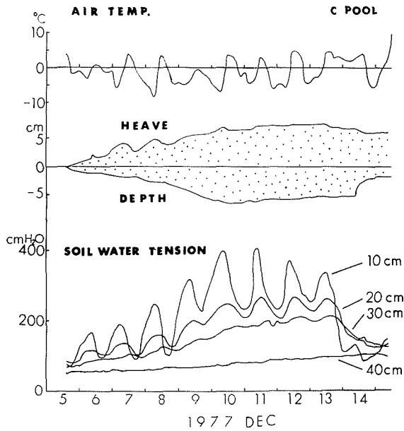
第1図 水分張力の日変化 (C プール)
