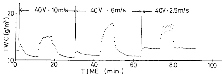
第9図 人工霧を与えたときの全含水量 (TWC) のヒーター電圧と管内風速に対する関係
