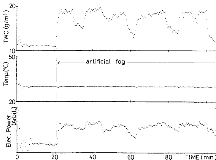
第10図 測定中の気温が一定になるようにしたときの TWC, 加熱温度, ヒーター電力の時間変化
