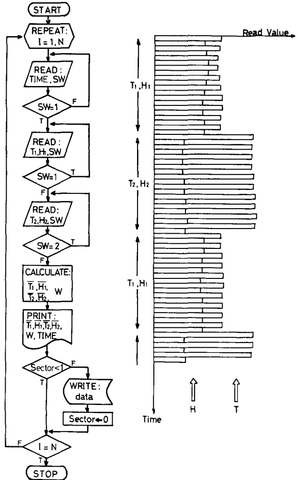
第2図 測定のプログラムとそのフローチャート センサー1とセンサー2を1秒間隔でそれぞれ10秒間測定し、その平均値よりLWCを求め、プリンターに出力する。
