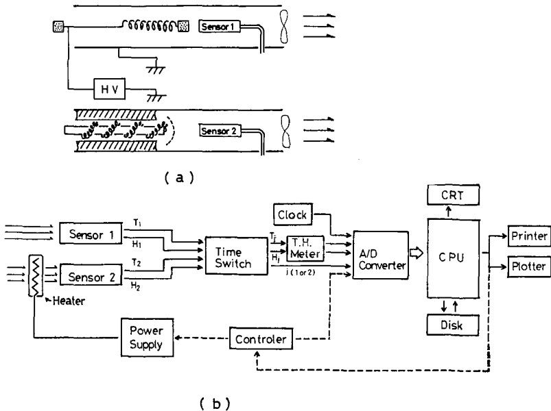
第1図 LWC TWC 測定システム
