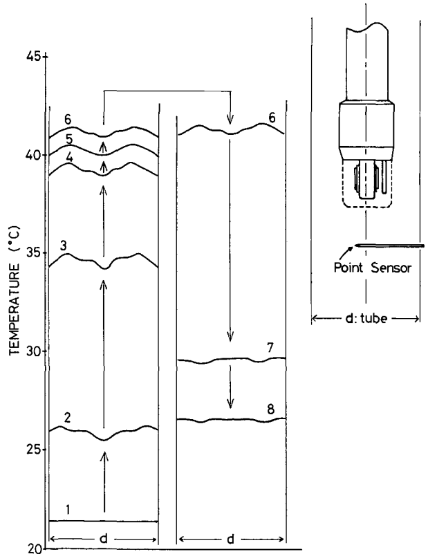
第6図 管内の温度分布の時間変化
