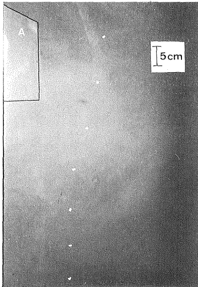
第2図 第1図と同じ。但し、雪片は破碎せず、プラスチック板(A)の方にひきつけられている
