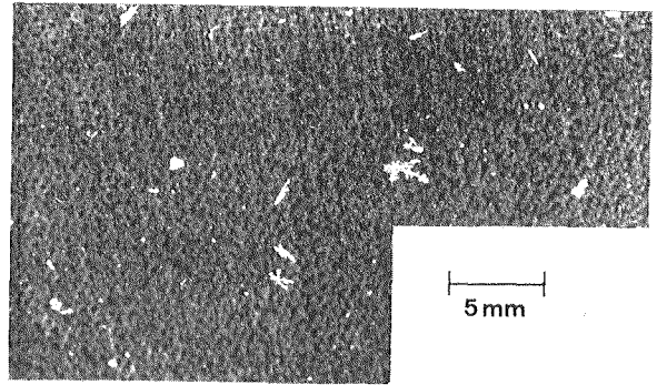
第3図 破碎した雪片の接写写真
