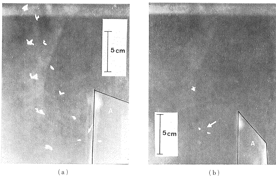
第1図 (a), (b) 落下中の雪片のストロボ写真。照明間隔は1/30秒である。図中矢印は、摩擦帯電したプラスチック板(A)の近傍を雪片が通過した際に、雪片が破碎したことを示している。雪片は、コントラストをつけるため、白く塗ってある
