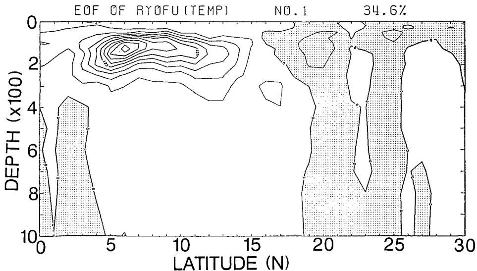
第2図 東経137度線の鉛直断面の海水温の EOF 第1成分の空間分布。ハッチは負の領域を示す
