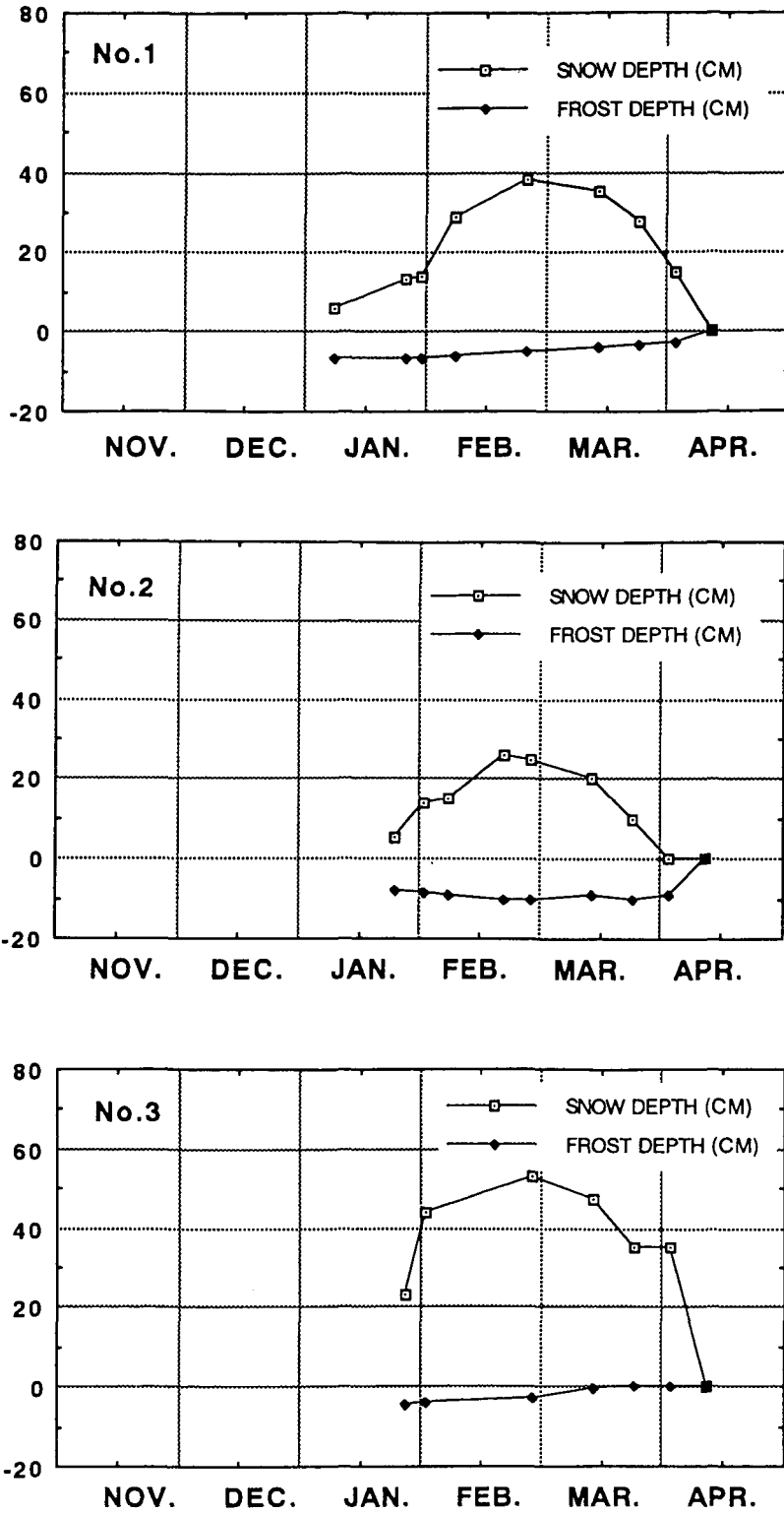
第 6 図 1990-91年冬の積雪深と凍結深の観測結果
