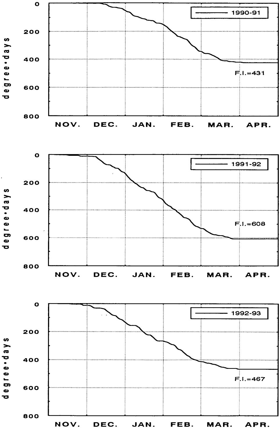
第3図 積算寒度の経時変化
