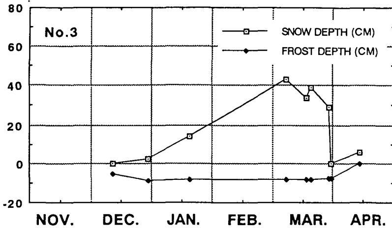
第7図 1991-92年冬期の積雪深と凍結深の観測結果
