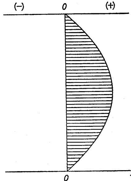
図-2 半径応力の理論的分布 Fig. 2. Theoretical distribution of radial stresses.
