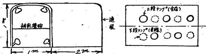
第2図 乾燥装置と赤外線ランプ配置図
