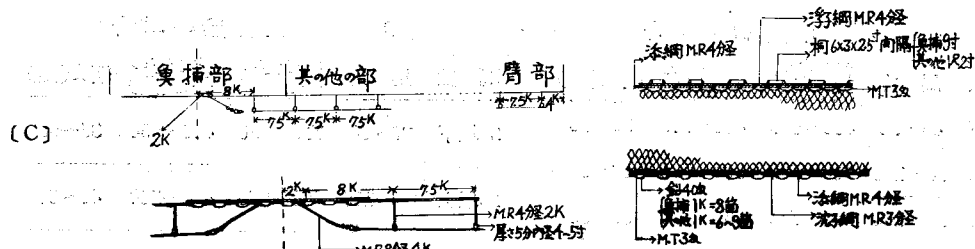
第1図 鯖揚繰網設計図 (K=間)
