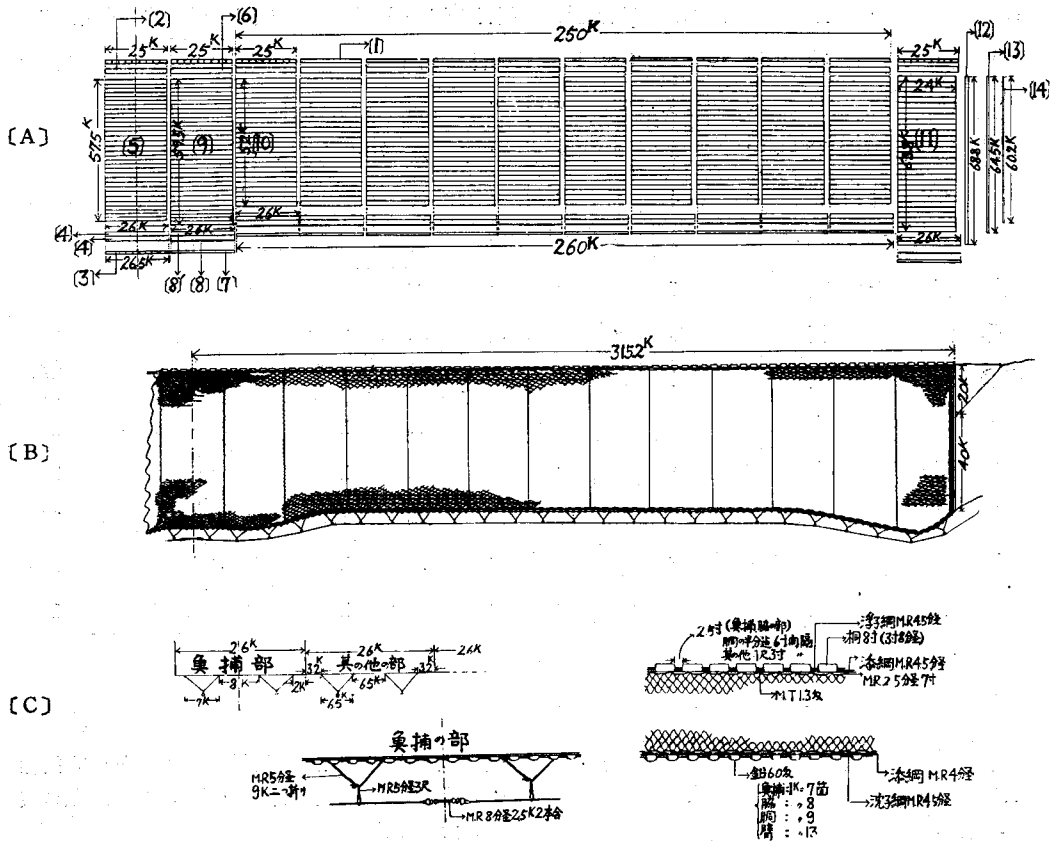
第2図 鯖巾着網設計図 (K=間)
