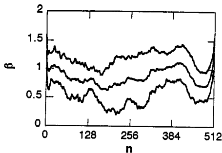
図5 512個のピッチ同期的な波形ゆらぎの周波数特性を 1/f^\beta 特性として近似するときの \beta の値の平均と標準偏差
