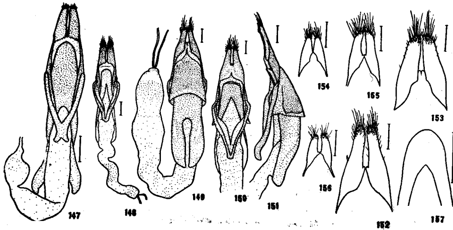
Fig. 147. Plectrura (Phlyctidola) metallica . Ventral view. Fig. 148. Psacotheta hilaris . Ventral view. Figs. 149-152. Monochamus rosenmülleri . Fig. 149. Dorsal view. Fig. 150. Ventral view. Fig. 151. Lateral view. Fig. 152. Dorsal view of lateral lobes. Figs. 153-156. Lateral lobes of Monochamus . All dorsal view. Fig. 153. Monochamus grandis . Fig. 154. M. tessarula . Fig. 155. M. saltuarius . Fig. 156. M. beloni . Fig. 157. Median lobe of Monochamus beloni . Ventral view.
