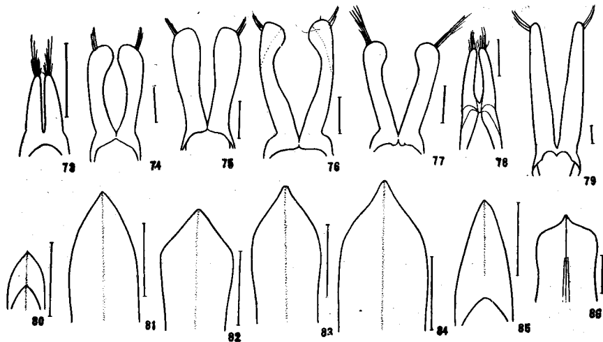
Figs. 73-79. Lateral lobes of Strangalia . All dorsal view. Fig. 73. Strangalia ( Pedostrangalia ) xanthoma . Fig. 74. Strangalia ( Strangalia ) arcuata f. mimica . Fig. 75. S. ( S. ) aethiops . Fig. 76. S. ( S. ) latipennis . Fig. 77. S. ( S. ) ochraceofasciata . Fig. 78. S. ( S. ) vicaria . Fig. 79. S. ( S. ) regalis . Figs. 80-86. Apical part of median lobe of Strangalia . All ventral view. Fig. 80. Strangalia ( Pedostrangalia ) xanthoma . Fig. 81. Strangalia ( Strangalia ) arcuata f. mimica . Fig. 82. S. ( S. ) aethiops . Fig. 83. S. ( S. ) latipennis . Fig. 84. S. ( S. ) ochraceofasciata . Fig. 85. S. ( S. ) vicaria . Fig. 86. S. ( S. ) regalis .
