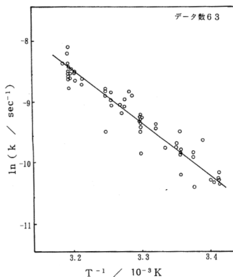
Fig. 2 改良した実験の結果(酢酸メチルの塩酸触媒加水分解反応のArrheniusプロット)
