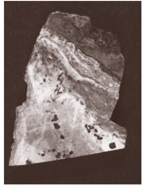
新鉱物Natropopphyllite ソーダ魚眼石
