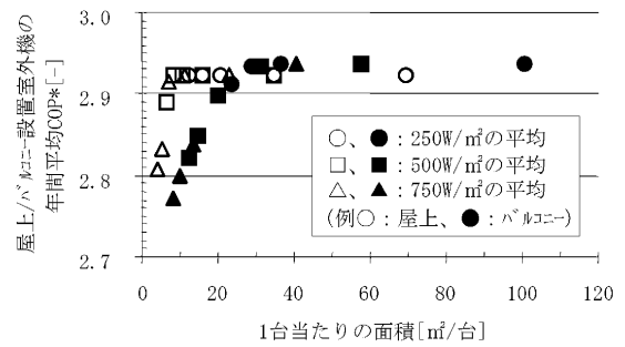
図 3 空調機の年間平均 COP*
