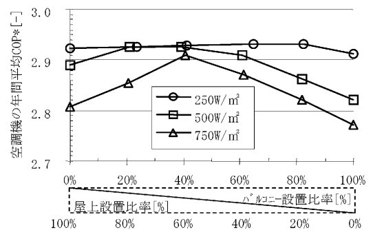
図 4 室外機の設置比率と空調機の年間平均 COP*
