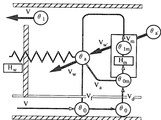
図2 室内空気再循環気流方式のモデル 二重床吹出し・横吹込み方式の場合
