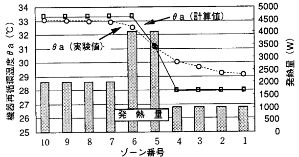
図4 実験値と計算値（ケースB-1）
