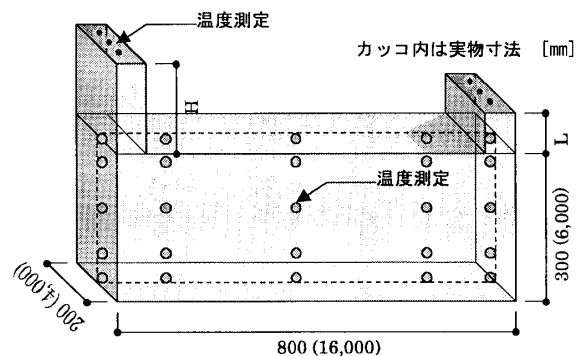
図2 模型図
