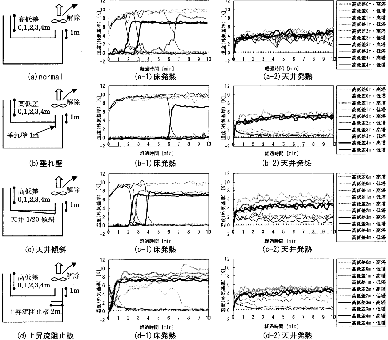
図3 吸引停止後の温度変化
