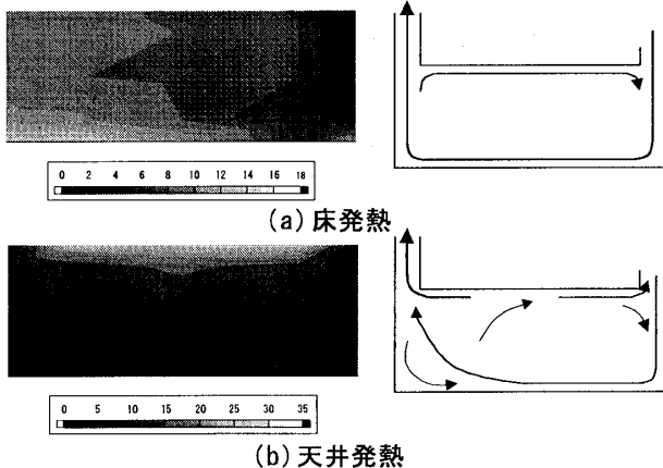
図4 温度分布と流れ(normal・高低差2m)
