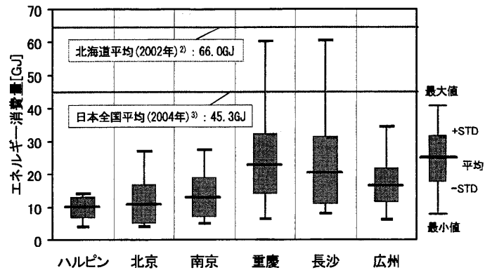
図-4 各都市の年間エネルギー消費量と日本の比較
