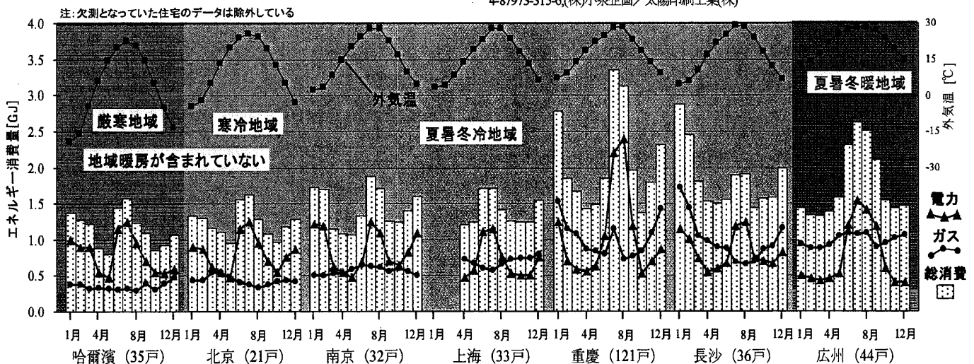
図-5 月別エネルギー消費量と外気温
