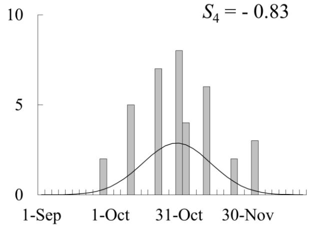
(d) Synchrony, 20 females
