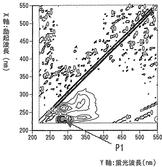
図7 風呂用洗剤の三次元励起・蛍光スペクトル図
