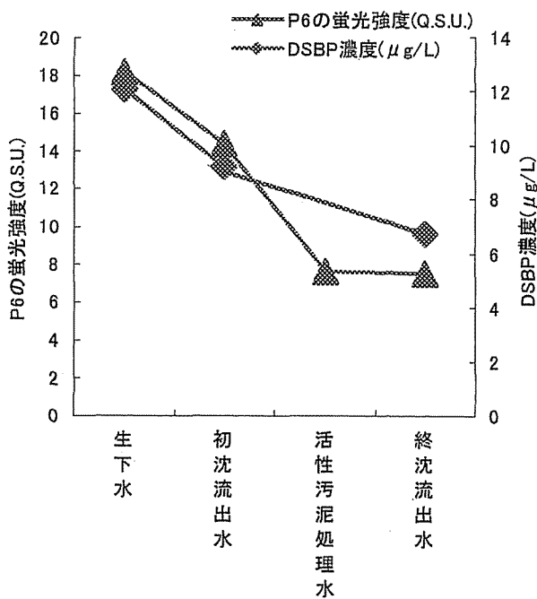
図5 下水処理過程における蛍光増白剤の蛍光強度変化 (DSBP は文献値)
