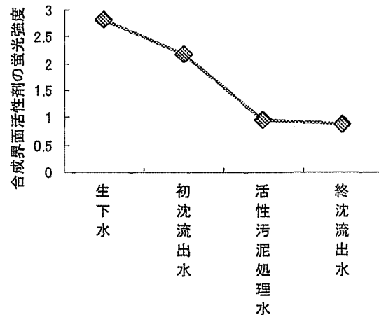
図9 下水処理過程における合成界面活性剤の蛍光強度変化
