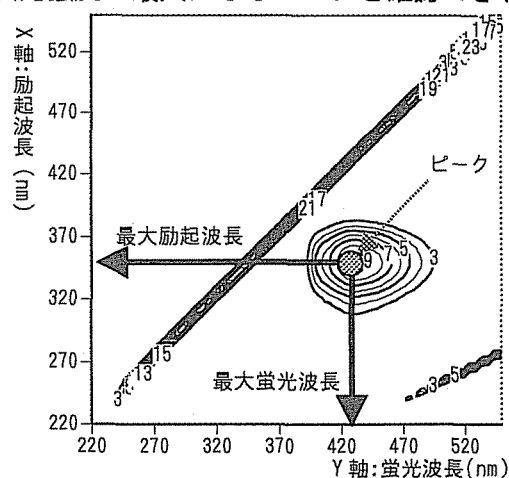
図1 三次元励起・蛍光スペクトル図
