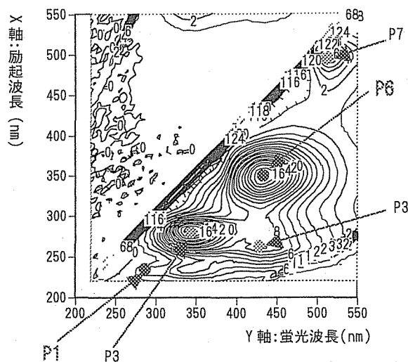
図2 生下水の三次元励起・蛍光スペクトル図と確認されたピーク
