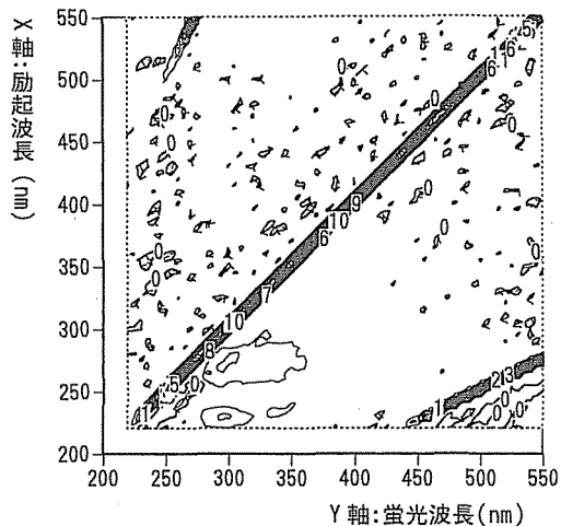
図3 蛍光増白剤無添加の洗濯用洗剤の三次元励起・蛍光スペクトル図
