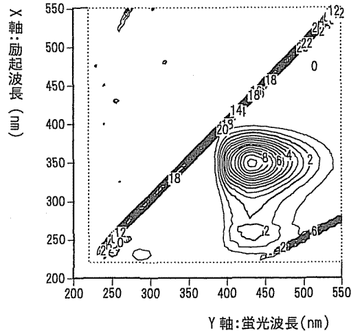
図4 蛍光増白剤添加の洗濯用洗剤の三次元励起・蛍光スペクトル図
