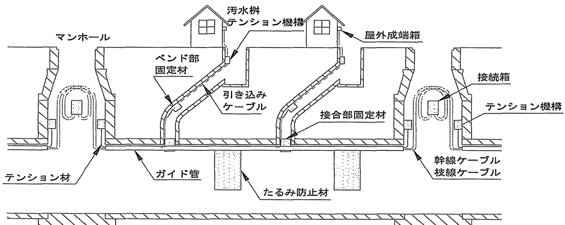
図1 テンションガイド工法敷設概要図
