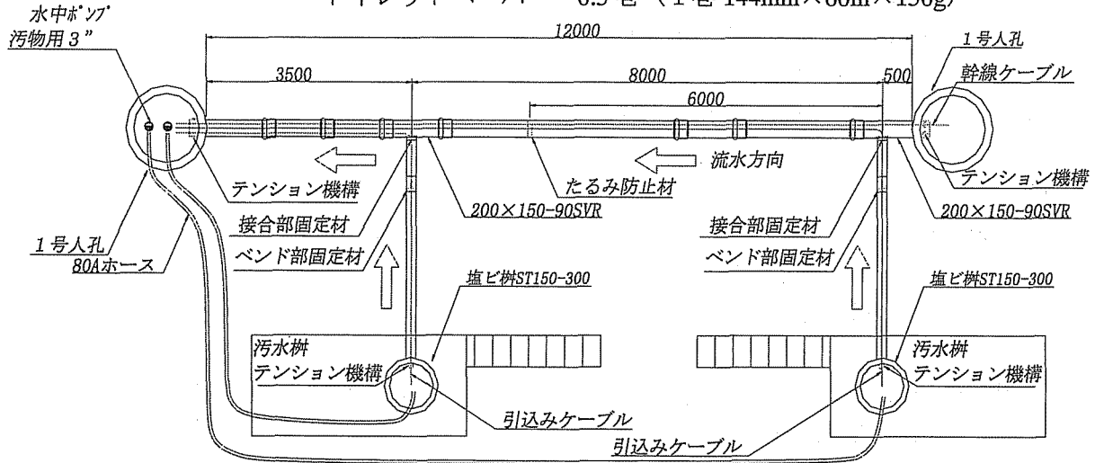
図 10 実験用管路
