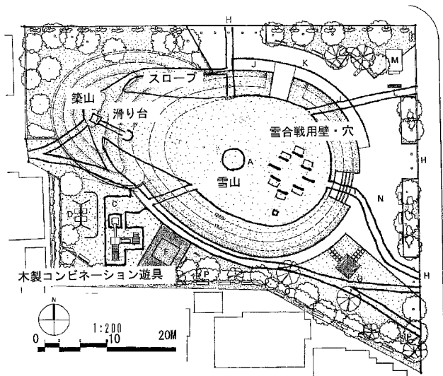
図6-2 北光公園平面図(整備後)
