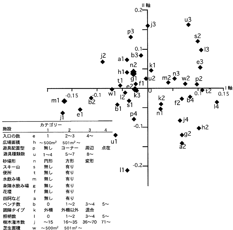
図2-3 街区公園の施設設置のパターン分析
