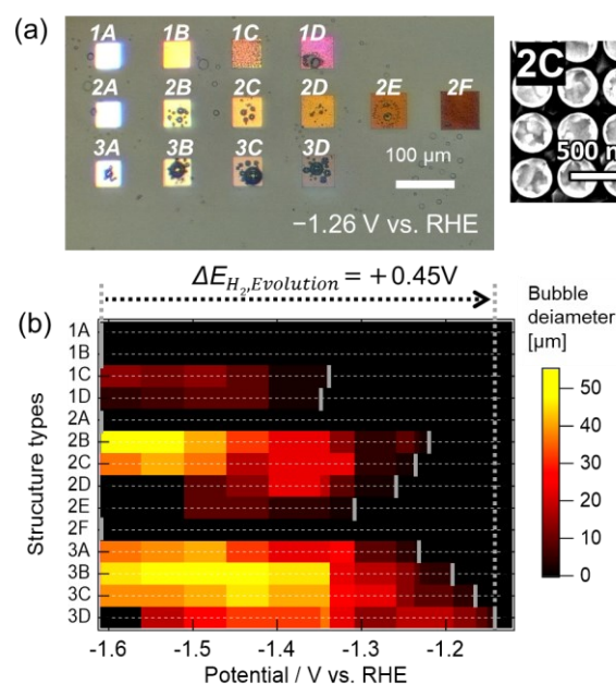
図1 (a)プラズモンモードが規定された銀ディスク正方格子の75MPa中0.5 MNaClO 4 水溶液中の-1.26 V RHEでの気泡発生光学像および一部構造のSEM像。(b)電位掃引による各格子構造と発生気泡の直径の相関。
