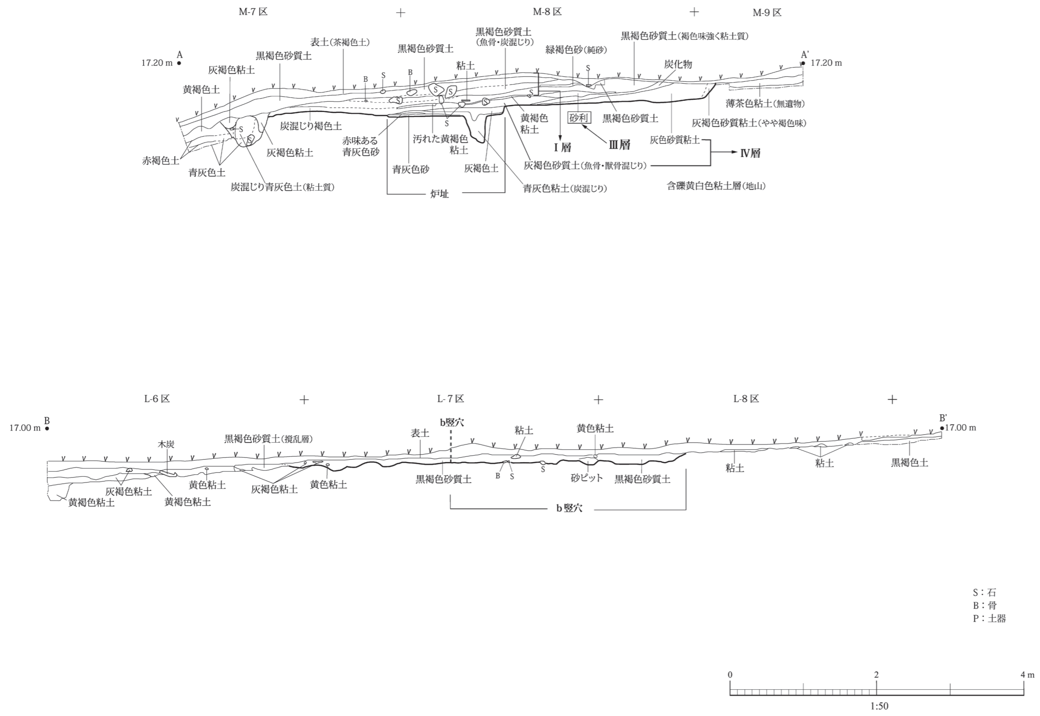
第2図 3号竪穴住居址土層断面図(1) A-A' (南北)・B-B' (南北)
