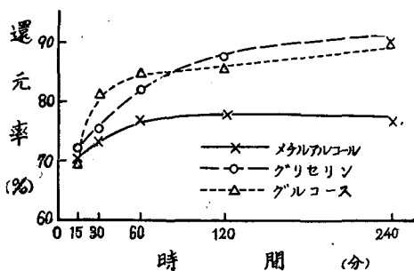
第 4 圖 時間と還元との關係 硫酸濃度 3.28 N 算定鹽基度 33.3% 沸騰點
