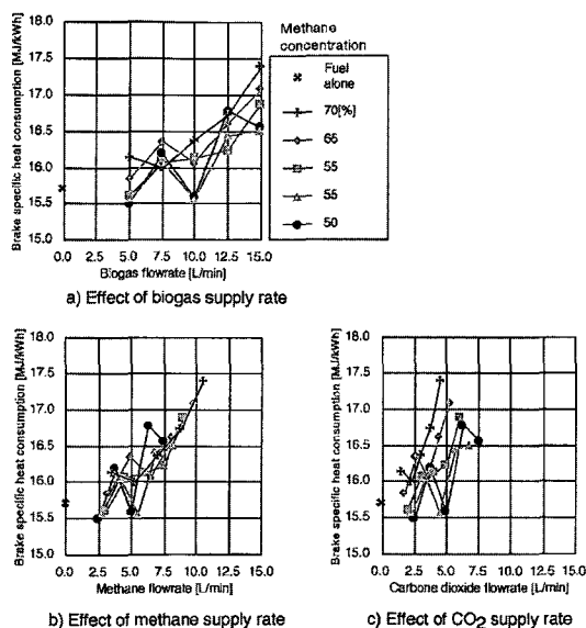
図3.1 ガス成分が熱消費率に与える影響
