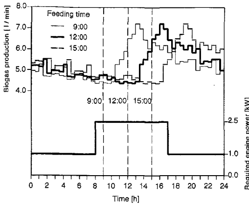
図4.3 ガス発生率と機関負荷の時間変動
