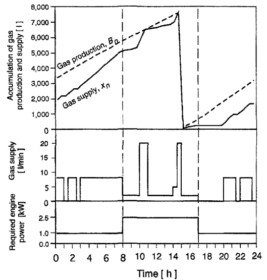
図4.7 煙濃度最小化の最適スケジュール
