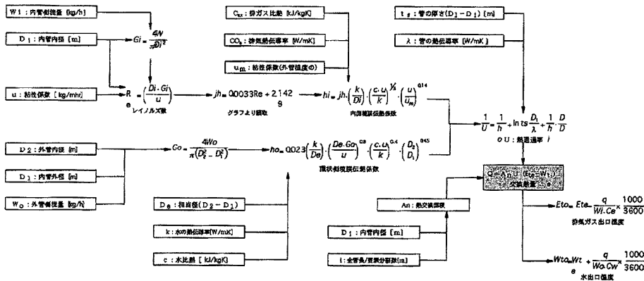
図6.3 交換熱量計算フロー Fig. 6.3 Heat exchange calculation flow
