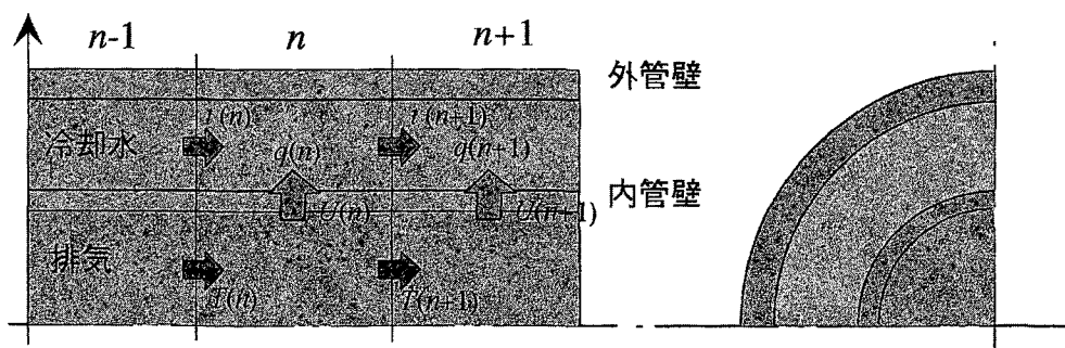
図6.2 排気熱交換器シミュレーションモデル
