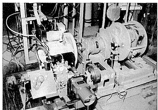
図2.5 供試機関全形
