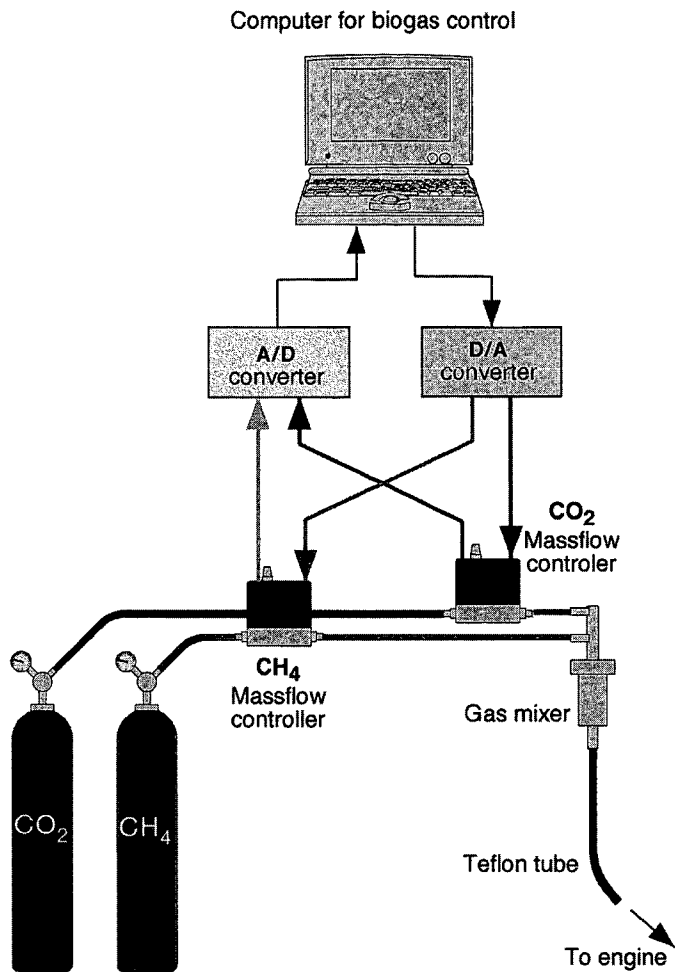
図2.4 バイオガス供給装置の構成 Fig. 2. 4 Construcion of biogas supplying apparatus
