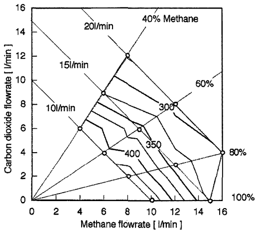
図3.16 ガス組成とNO x 濃度の関係
