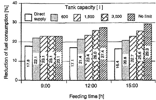
図4.4 最適化による軽油消費量の減少率
