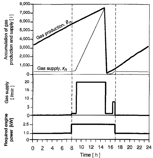
図4.5 軽油消費最小化のガス供給スケジュール
