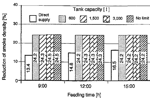
図4.6 最適化による煙濃度の減少率
