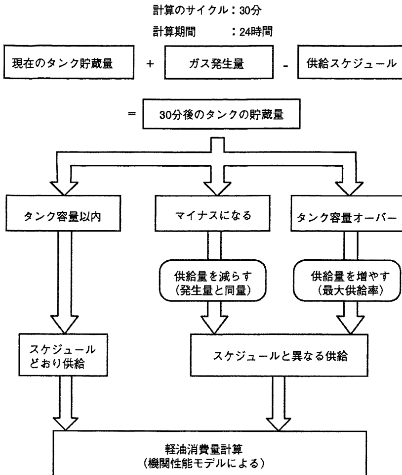
図5.1 シミュレーションのアルゴリズム
