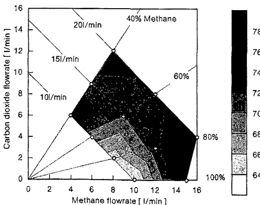
図3.17 ガス組成と煙濃度の関係
