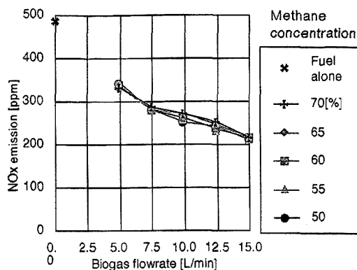
図3.3 NOx 濃度の変化 Fig. 3.3 Change of NOx emission
