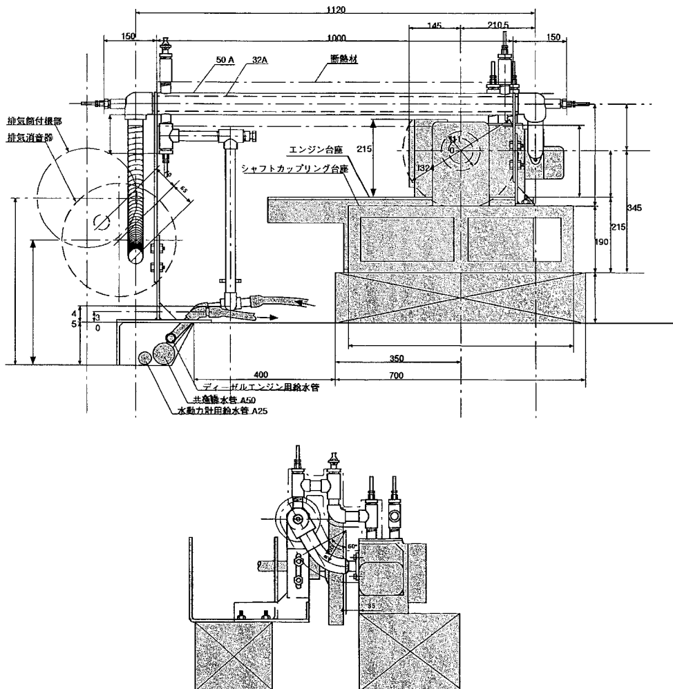
図6.4 熱交換器設計図
