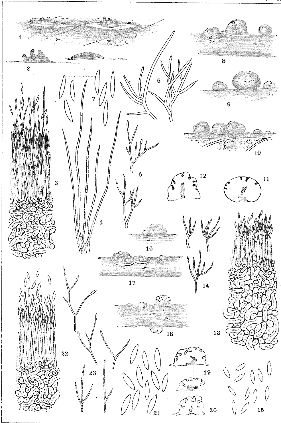
1—7. Aschersonia Aleyroides Webber. 8—15. A. marginata Ell. et Ev. 16—23. A. Suzukii Miyabe et Sawada.
