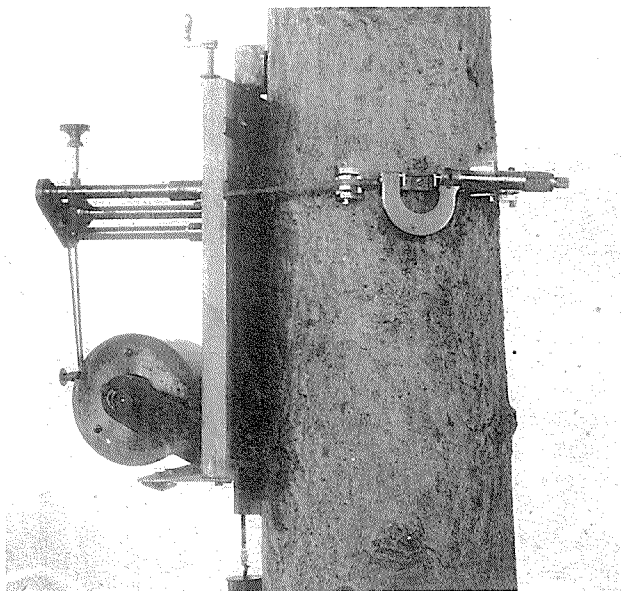
Abbildung III. Kontrollvorrichtung.
