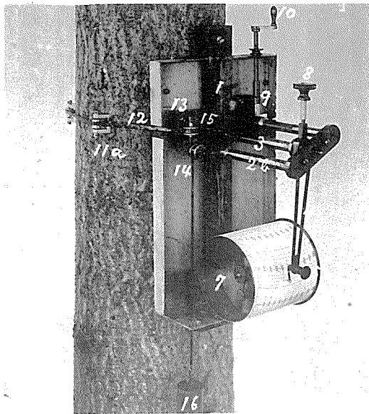
Abbildung II. Zuwachsaufograph.
