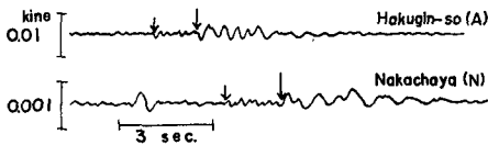
第17図 火山性微動(B'-型地震)の記録の一例(7月6日, 6時頃)
