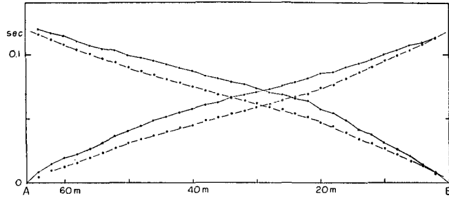
第11図 初動の走時(●)及び T' (○)
