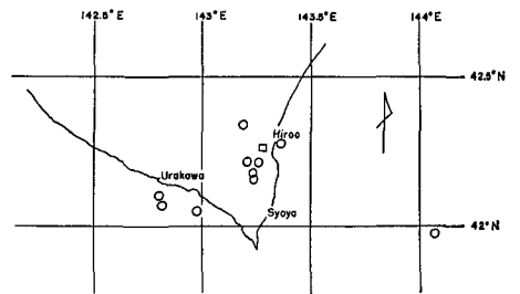
第9図 4点観測から求められた震央分布 Fig. 9. Epicenters determined by the quadruple sets of observations, \circ ; h < 100 km, \square ; h > 100 km.
