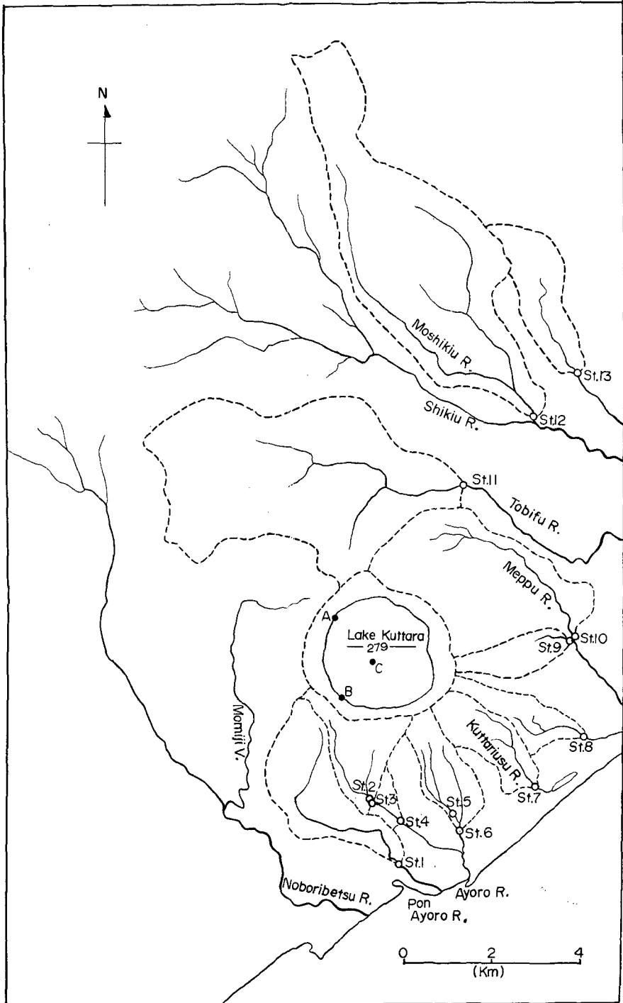
第7図 倶多楽湖周辺の河川流域の概略
