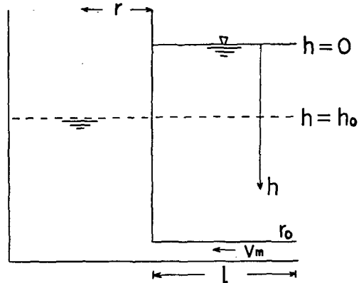
第 2 図 湖或いはプールの水位変化に伴う水位計の測定水面の変化
