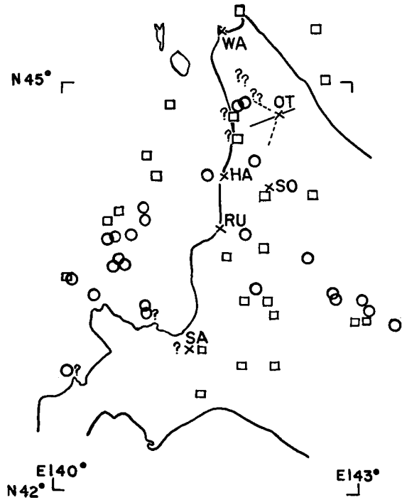
第 5 図 道北地方における震央分布
