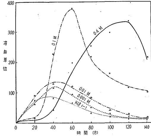
図7 KCl濃度と毒素産生との関係
