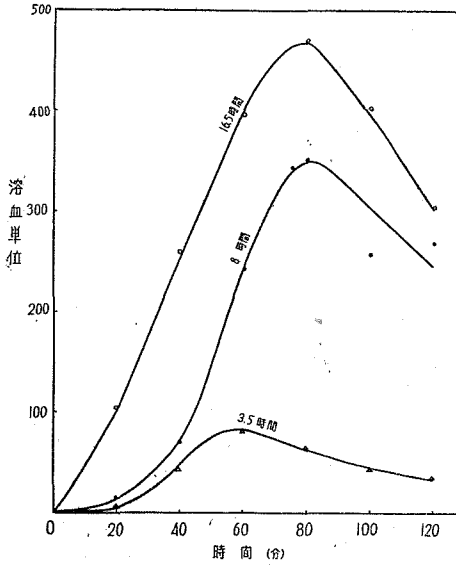
図1. 菌体の発育期と毒素産生能との関係 培養時間 3.5時間, 8時間, 16.5時間の菌体は3回洗滌後に磷酸緩衝液加食塩水(pH 7.0)を用いて約20 mg/mlに浮遊させたものを菌液とした。 反応液: 菌液 0.75 ml, RNA (200 μg/ml) 0.15 ml, 0.05 M maltose 0.15 ml, 0.02 M MgSO 4 0.15 ml, 0.5 M KCl 0.3 ml, (全量 1.5 ml)。
