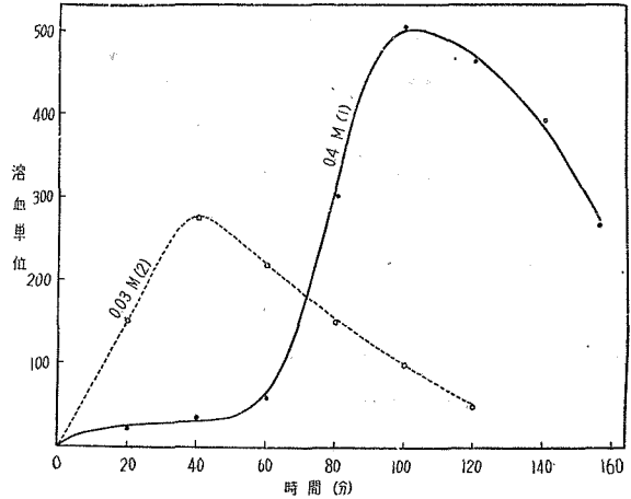
図 8. 毒素産生過程に及ぼす \text{KCl} 濃度の影響 (1)
