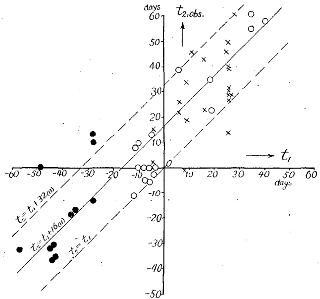
第3圖 時間原点から凍結初日までの日数 t_{2,obs} と気温が海水の凍結温度に降下するまでの日数 t_1 との関係 (黒丸：北極海、白丸：オホック海及びアムール灣、掛印：日本海)
