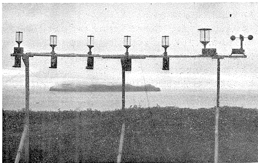
写真2 捕捉装置の配置 (1956年7月)
