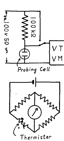
Fig. 2. Salinometer Circuit.
